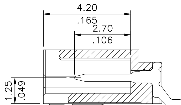
SEC. A-A
